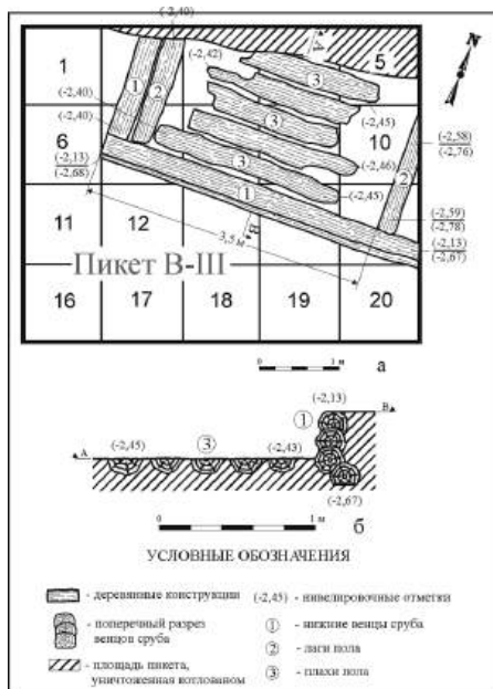
Рис. 8. Сооружение 5: а — планиграфия, б — поперечный разрез
