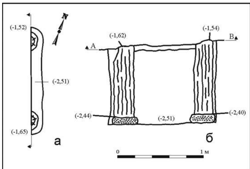
Рис. 4. Подвал сруба-пятистенка: а — планиграфия, б — поперечный разрез
