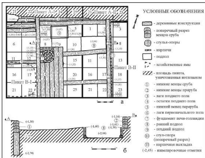
Рис. 3. Сооружение 1: а — планиграфия, б — поперечный разрез
